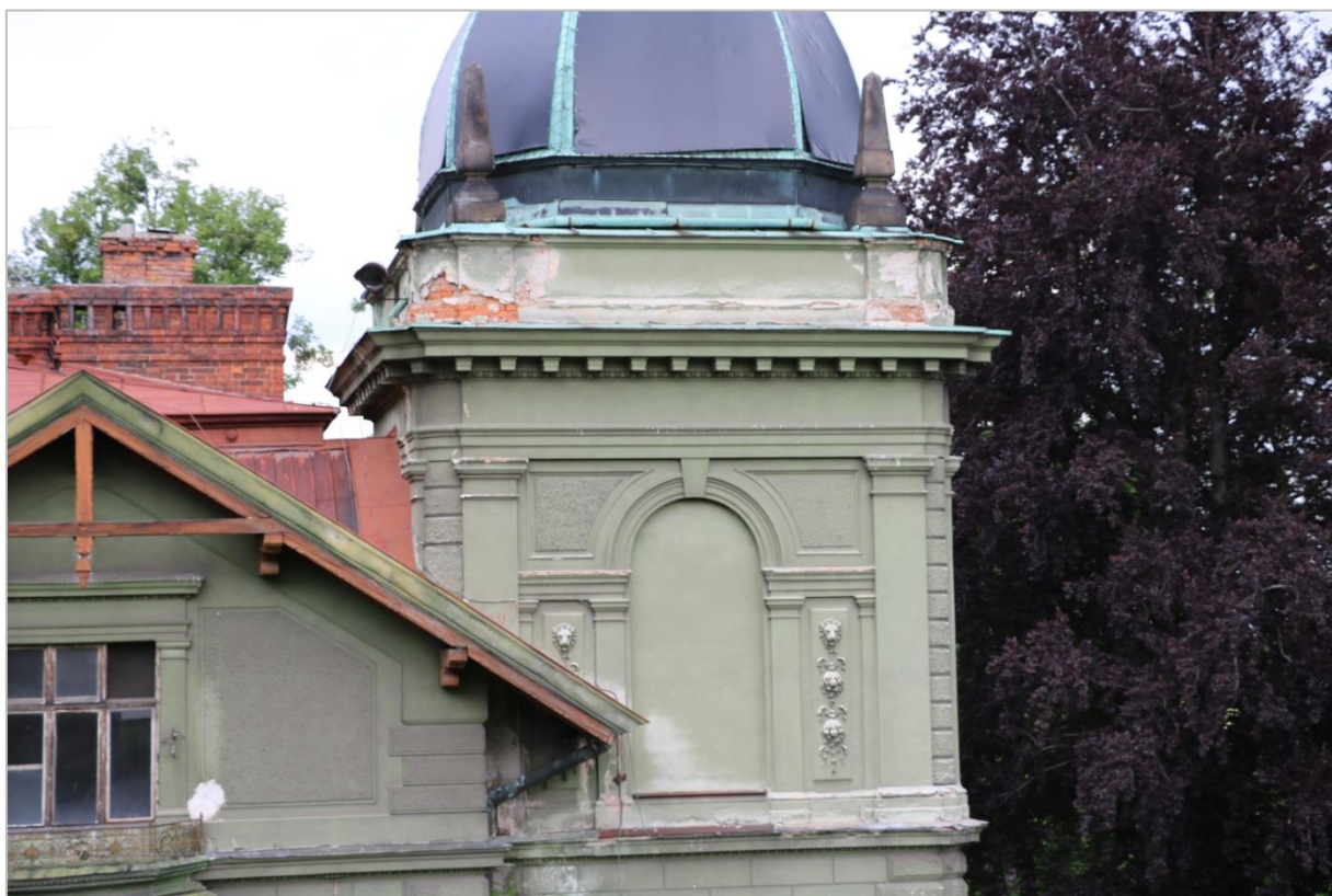
Zazděné okno ve věž , poškozená omítka, oplachtovaná báň
