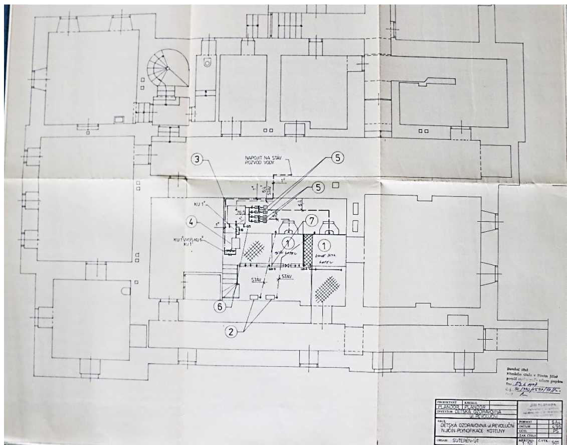
Plán na úpravu kotelny, Plandor J., 1996-7
