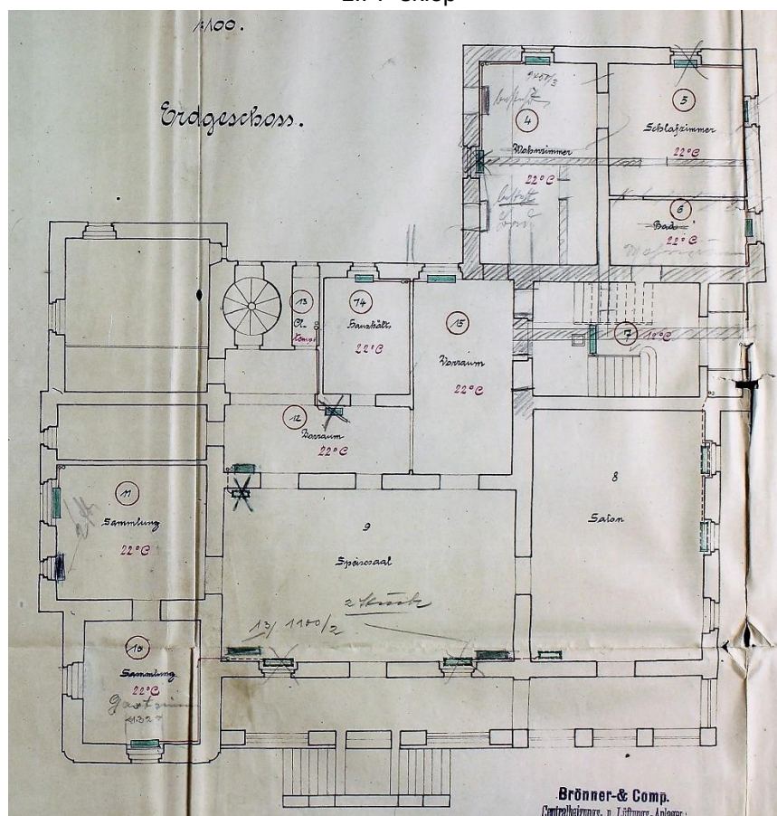
1.NP se slabou viditelnou kresbou skutečného stavu přístavby
